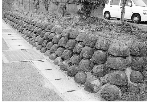
写真 1；帯江鉾山の鉾滓（鰯：カラミ）を利用したのり面（2007 年 4 月）
